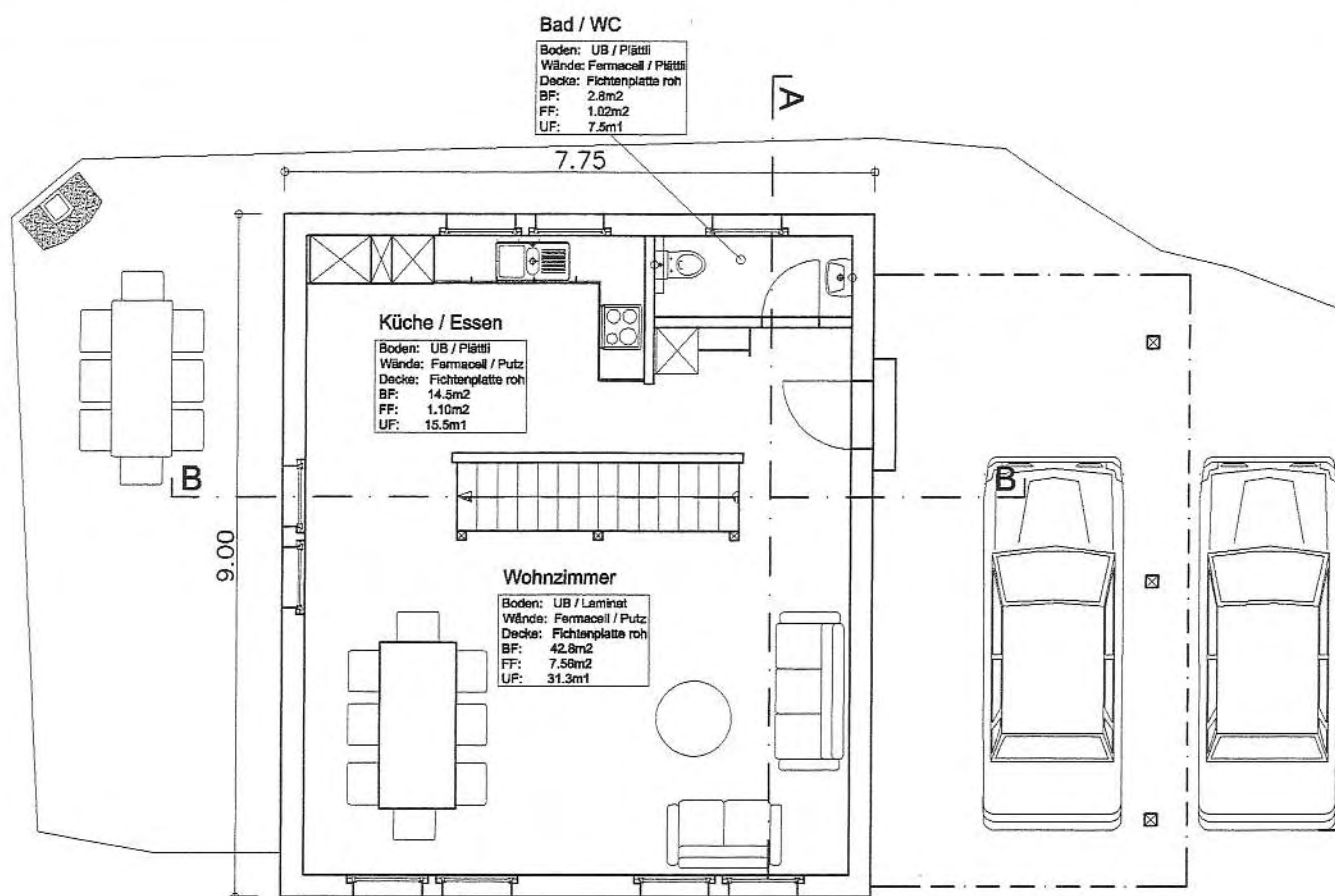
Grundriss Erdgeschoss
