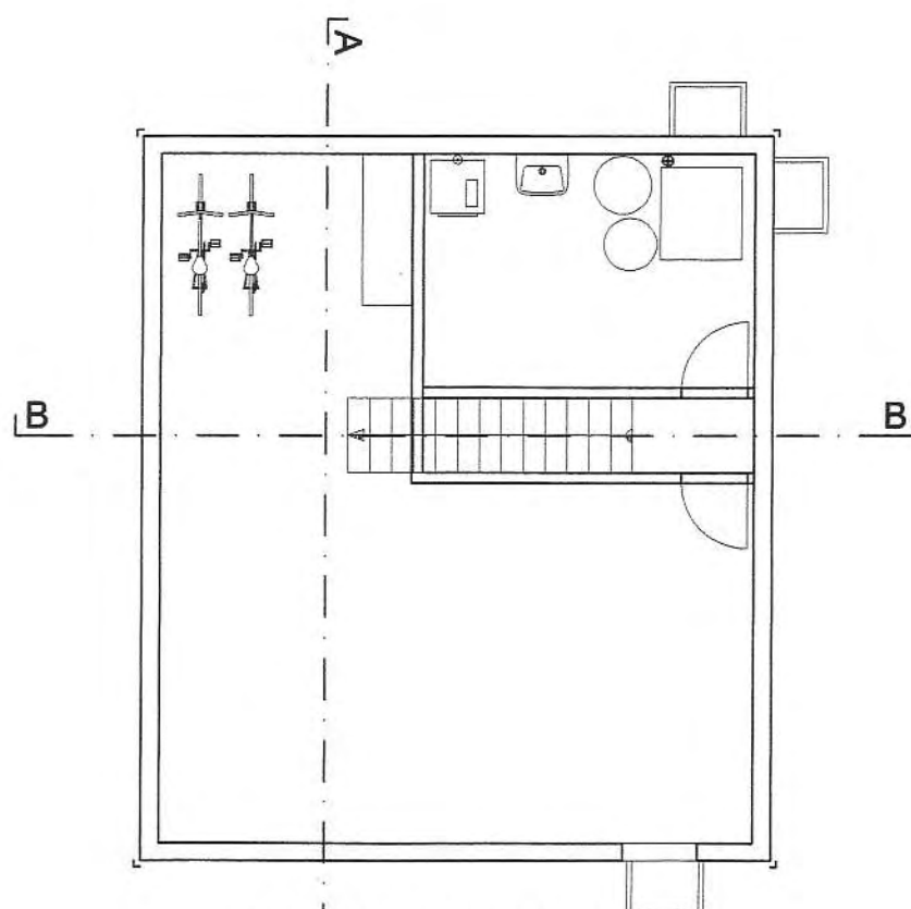
Grundriss Untergeschoss
